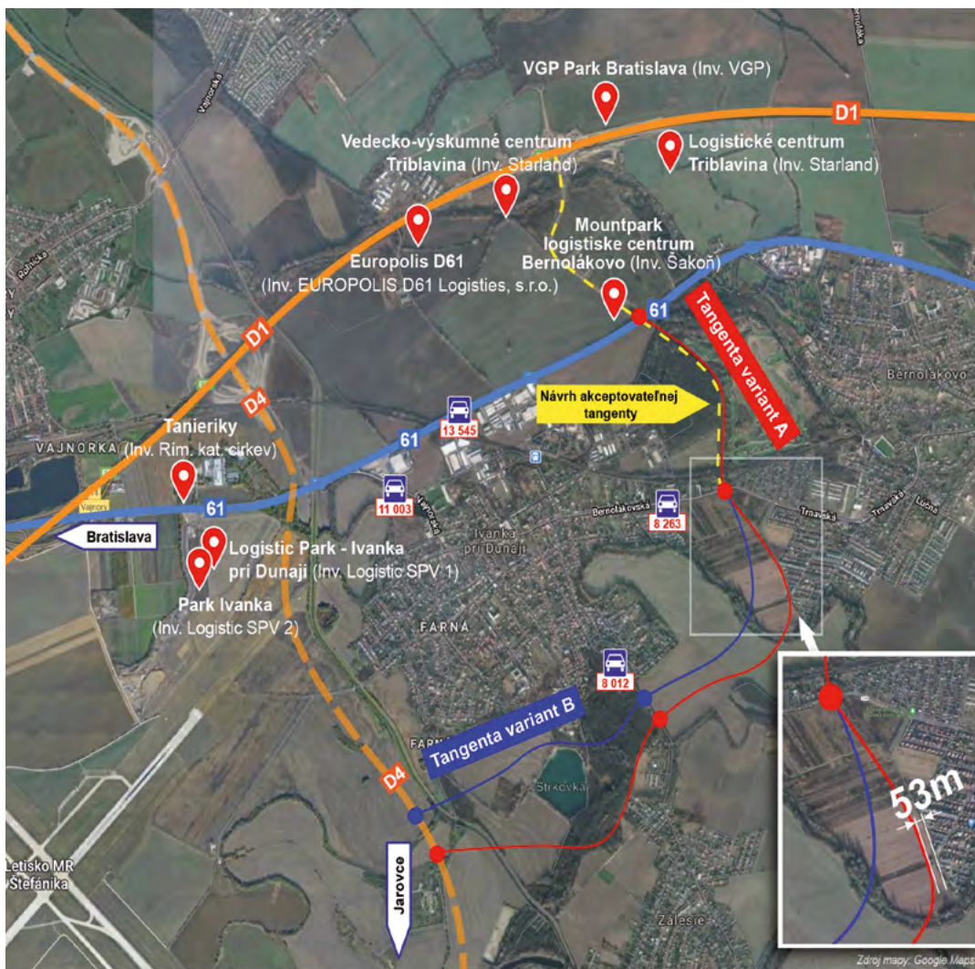
Podkladom na vyhotovenie náčrtu tangenty je technická štúdia Prepojenie ciest I-61 a D4
